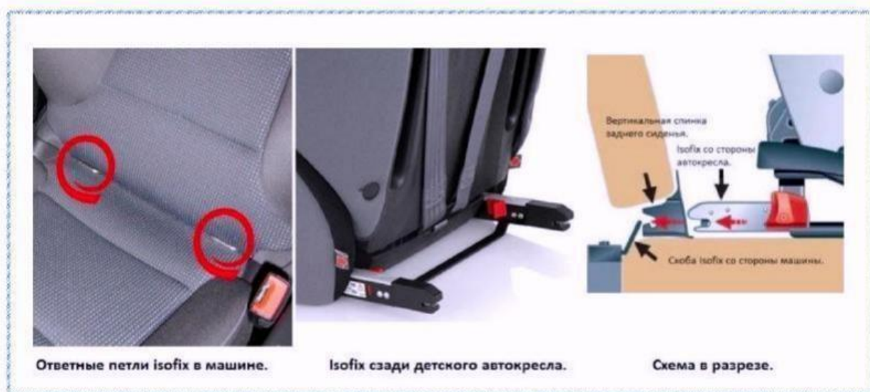
Рисунок 5. Крепления ISOFIX
